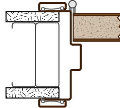
Jamb Hinge Side
