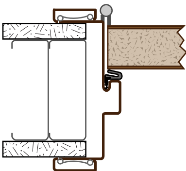
3A Jamb Hinge Side - Kerfed
