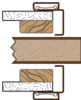
6A Jamb - Pocket Door Trim
